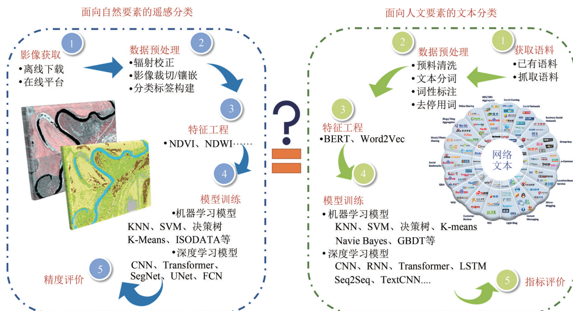
图 2 遥感影像和网络文本分类主要流程
