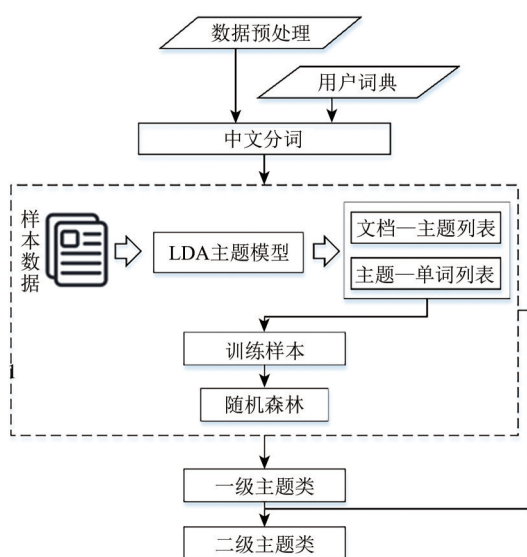
图5 主题抽取与情感分类框架
