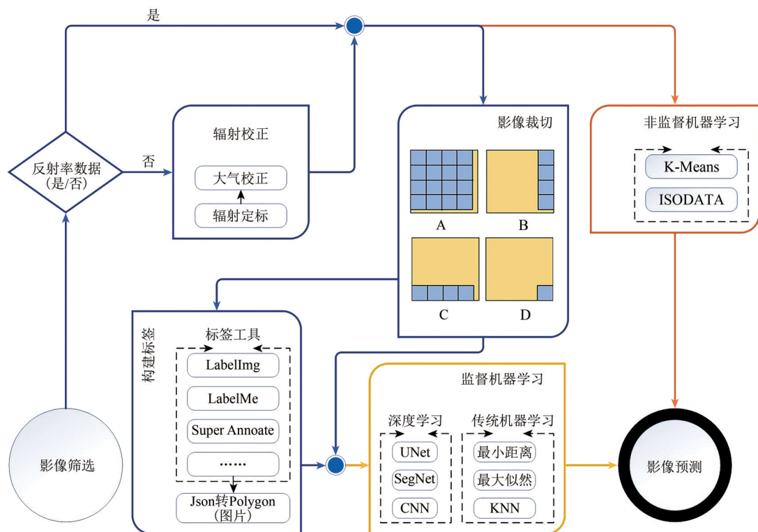
图3 水体提取技术路线
