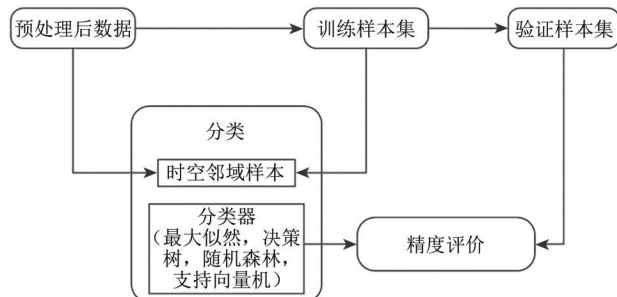
图4 土地覆盖分类技术路线
